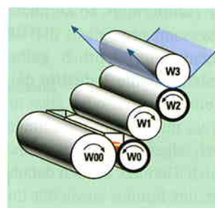
5-Walzenauftragungssystem
